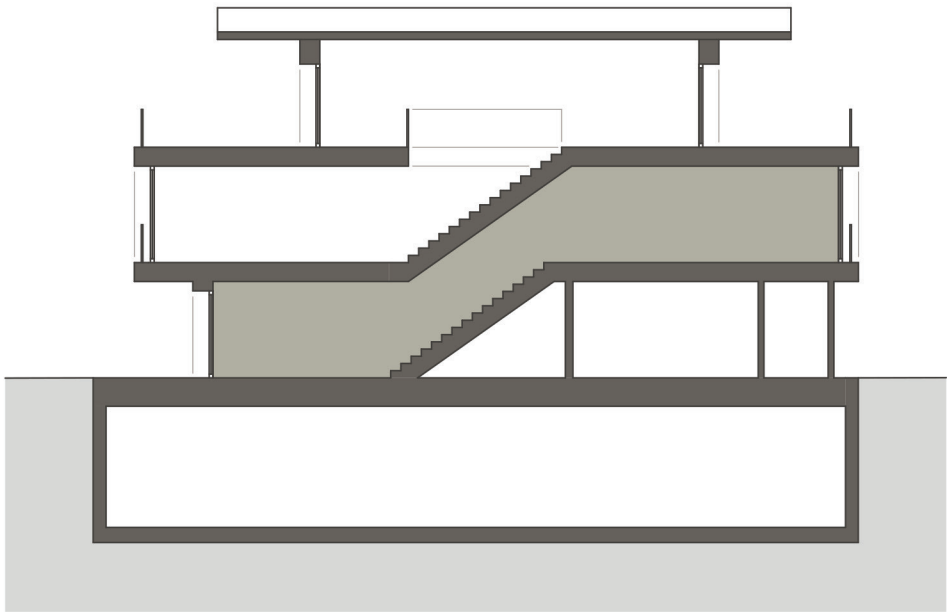
GEBÄUDESCHNITT
